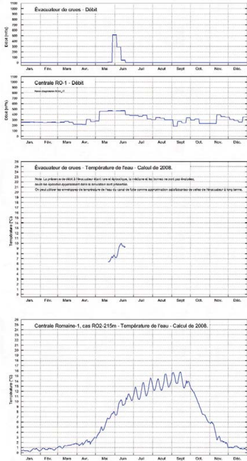
Planche 18. Réservoir Romaine-1. Température de l'eau et débit aux exutoires. Extrait 17 de 21 - Année 1999.
