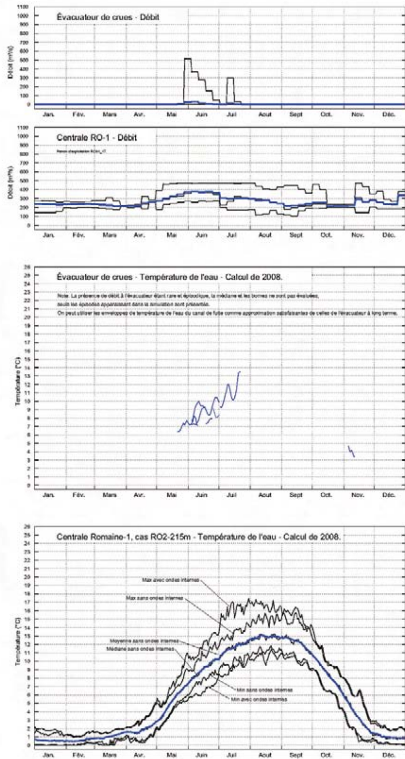
Planche 18. Réservoir Romaine-1. Température de l'eau et débit aux exutoires. Extrait 1 de 21 - Minima, maxima, médianes et moyennes.
