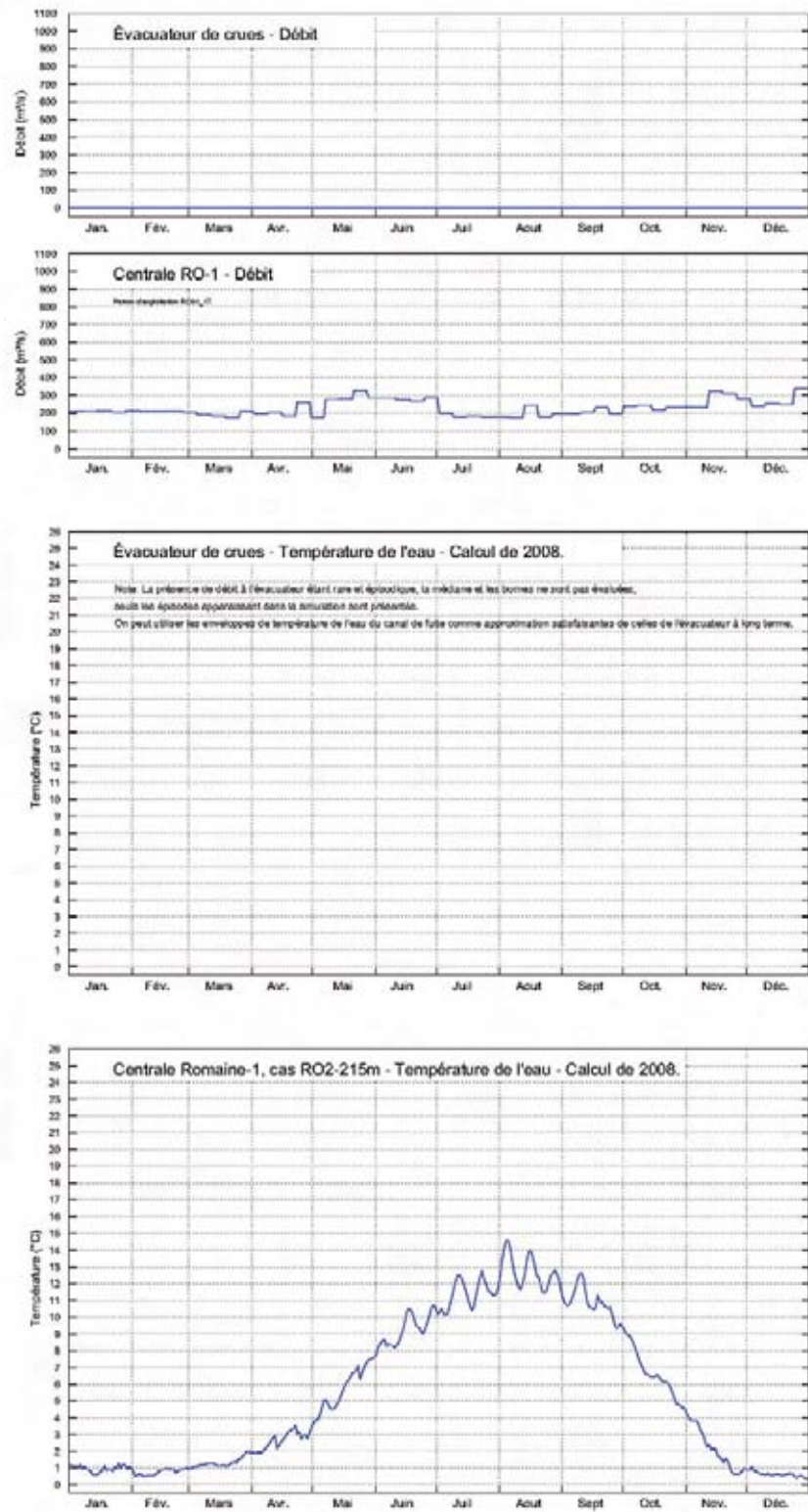
Planche 18. Réservoir Romaine-1. Température de l'eau et débit aux exutoires. Extrait 11 de 21 - Année 1993.
