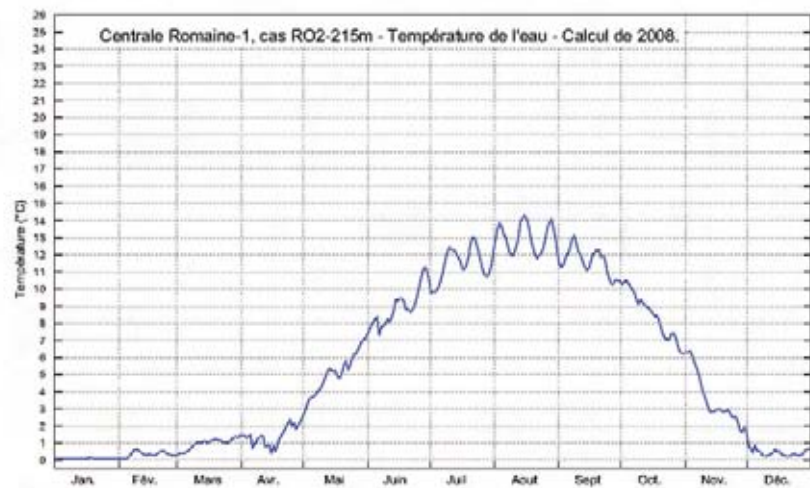
Planche 18. Réservoir Romaine-1. Température de l'eau et débit aux exutoires. Extrait 9 de 21 - Année 1991.
