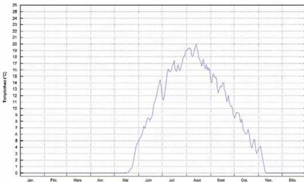
Rivière Romaine à l'état actuel. Température de l'eau au PK 16.
