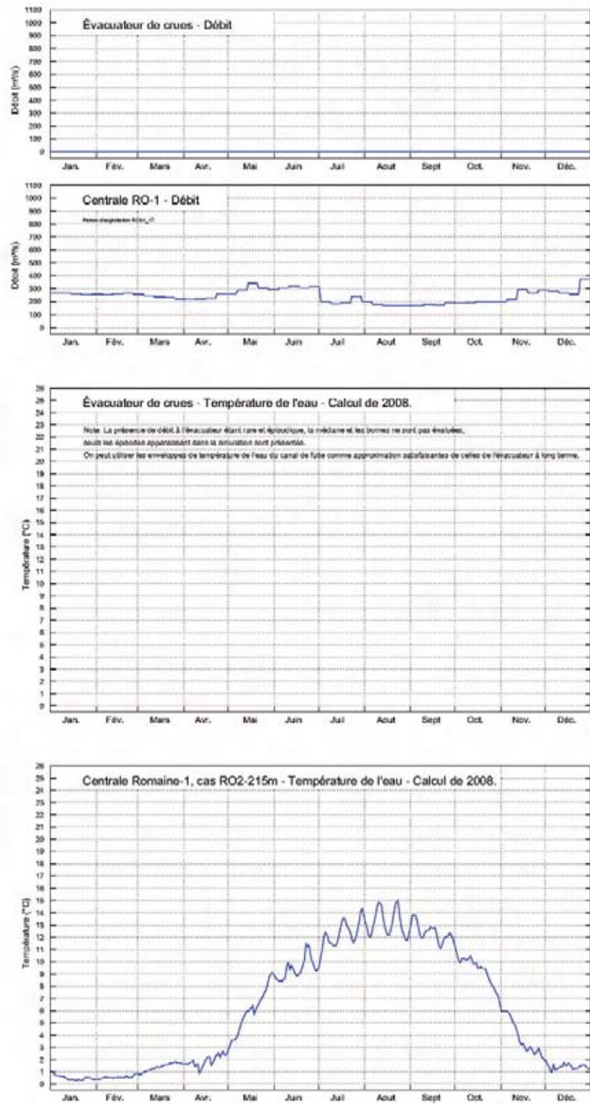
Planche 18. Réservoir Romaine-1. Température de l'eau et débit aux exutoires. Extrait 19 de 21 - Année 2001.
