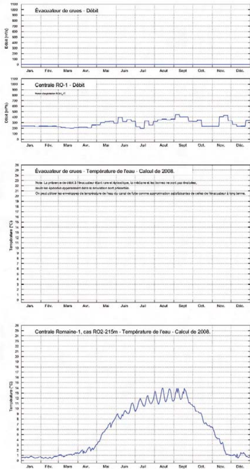
Planche 18. Réservoir Romaine-1. Température de l'eau et débit aux exutoires. Extrait 7 de 21 - Année 1989.
