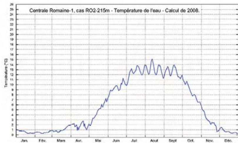
Planche 18. Réservoir Romaine-1. Température de l'eau et débit aux exutoires. Extrait 5 de 21 - Année 1987.
