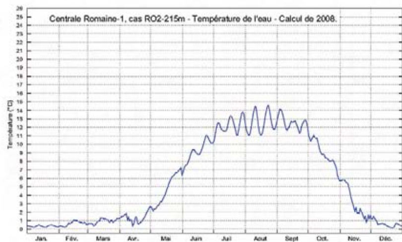
Planche 18. Réservoir Romaine-1. Température de l'eau et débit aux exutoires. Extrait 3 de 21 - Année 1985.
